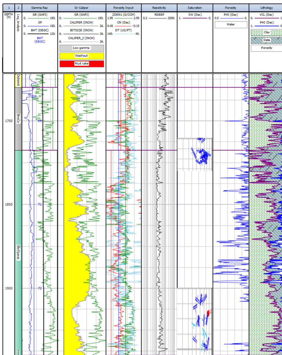
Slika 14: Karotažni dijagrami snimljeni u bušotini ZapGT-1 u intervalu breča i škriljavaca
