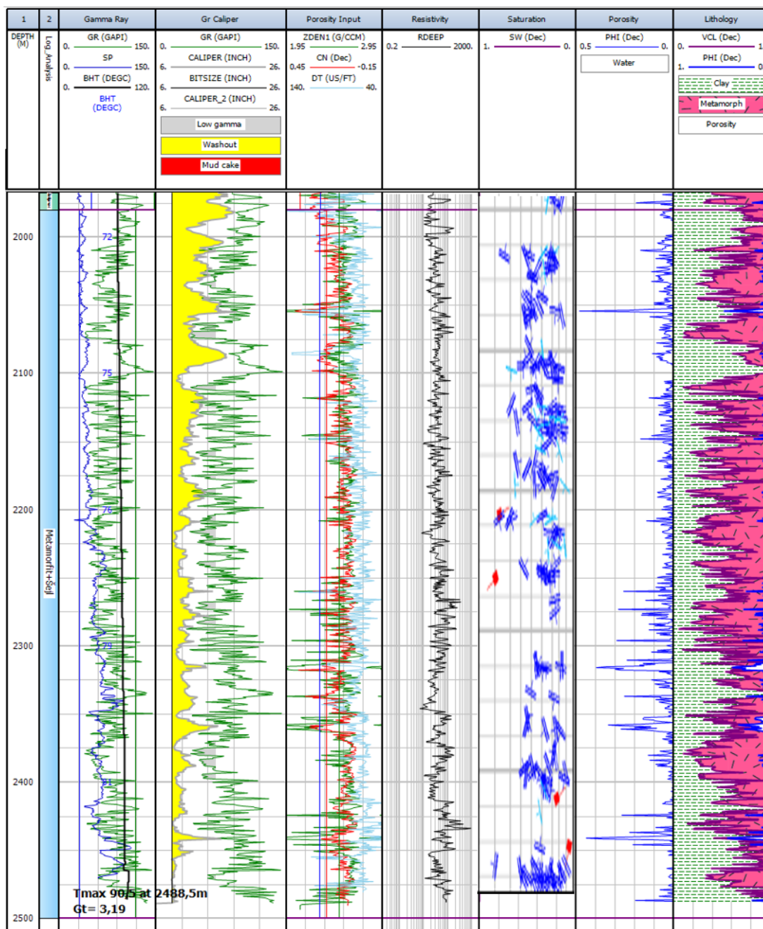
Slika 15: Karotažni dijagrami snimljeni u bušotini ZapGT-1 u intervalu metamorfita
