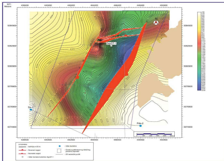
Slika 8 Dubinska strukturna karta po krovini EK markera Pn
