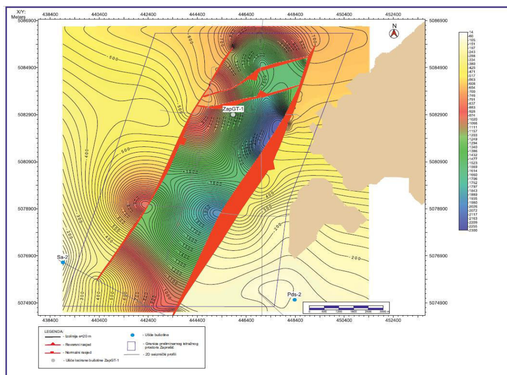
Slika 7 Dubinska strukturna karta po krovini EK markera Rs7
