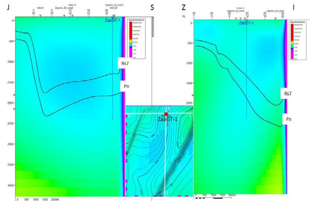
Slika 9 Poprečni i uzdužni profil iz 3D magnetotelurskog modela preko predložene bušotine ZapGT-1
