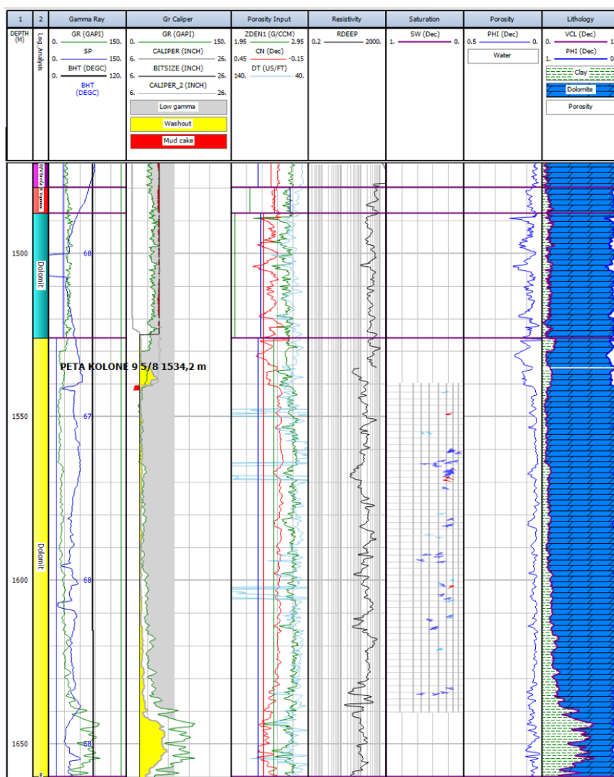
Slika 13: Karotažni dijagrami snimljeni u bušotini ZapGT-1 u intervalu dolomita
